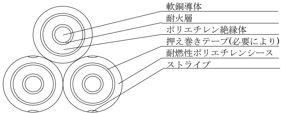
断面図
